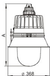
带灯伞(S)
