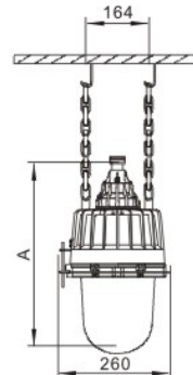
吊链式(D)
