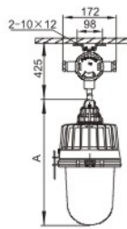
吊杆式(G)
