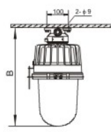
吸顶式(X)
