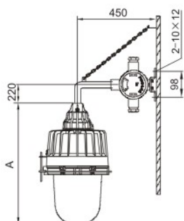
壁式(B2)90°
