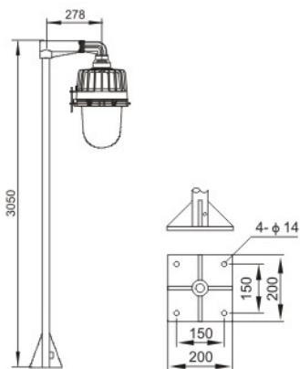
法兰式(F1)
