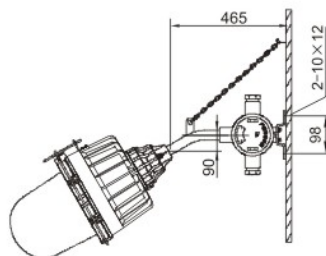
壁式(B1)30°
